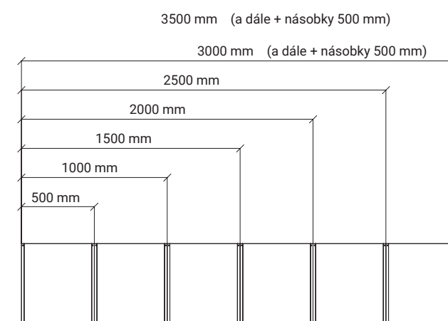
Rozměry rovných sestav skříní UNIVERSAL
