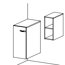
LN 11 skříňka závěsná hluboká, policová s dveřmi / 300 x 672 x 588 /
