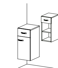
LN 04 skříňka závěsná mělká, policová s dveřmi a zásuvkou / 300 x 672 x 388 /
