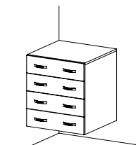
LN 18 skříňka závěsná hluboká, zásuvková / 600 x 672 x 588 /
