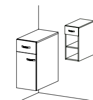
LN 13 skříňka závěsná hluboká, policová s dveřmi a zásuvkou / 300 x 672 x 588 /
