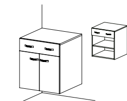
LN 17 skříňka policová s dveřmi a zásuvkou / 600 x 672 x 588 /
