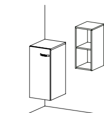
LN 01 skříňka závěsná mělká, policová s dveřmi / 300 x 672 x 388 /
