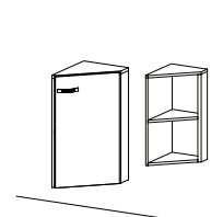
LN 10 skříňka závěsná mělká, policová s dveřmi rohová pravá / 300 x 672 x 388 /
