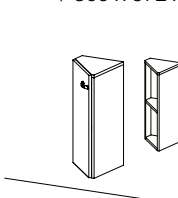
LN 09 skříňka závěsná mělká, policová s dveřmi rohová levá / 300 x 672 x 388 /
