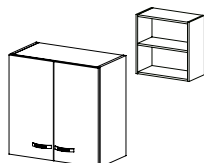
LN 27 skříňka závěsná horní, s dveřmi / 600 x 600 x 318 /
