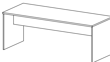
ST 97 stůl jednací / 2000 x 750 x 800 /
