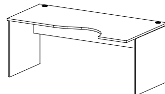
ST 73 stůl pracovní tvarový / 1800 x 750 x 1000/400 /
