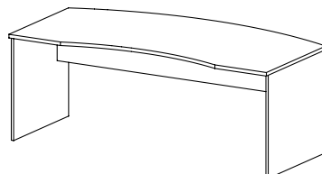
ST 81 stůl pracovní tvarový / 2000 x 750 x 1000/800 /
