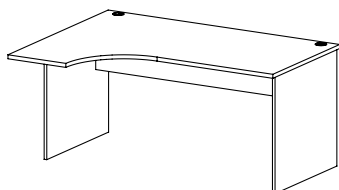
ST 78 stůl pracovní tvarový / 1600 x 750 x 1200/400 /
