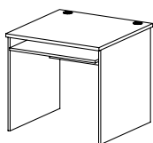
ST 31 stůl pod PC / 800 x 750 x 800 /
