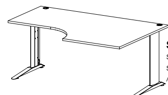
ST 64 stůl pracovní tvarový s kovovou podnoží / 1800 x 750 x 1200/800 /
