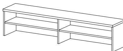
ST 35 pultová nástavba / 1600 x 350 x 320 /
