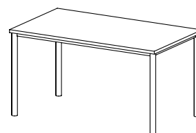
ST 48 stůl pracovní / 1400 x 750 x 800 /
