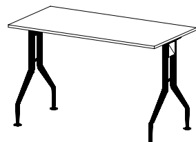
SL 204/18 SL 204/25 školní lavice / 1350 x 738 x 600 /
