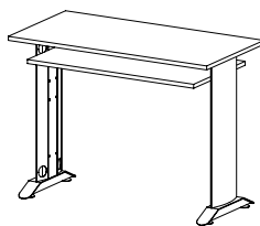
SL 106/18 SL 106/25 školní lavice s pevnou policí / 1000 x 738 x 500 /
