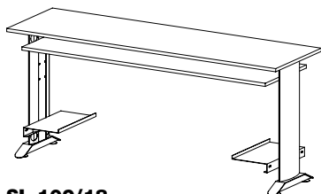
SL 109/18 SL 109/25 školní lavice s pevnou policí a držáky pro PC / 1700 x 738 x 500 /
