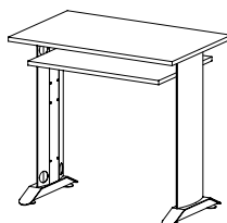
SL 105/18 SL 105/25 školní lavice s pevnou policí / 800 x 738 x 500 /
