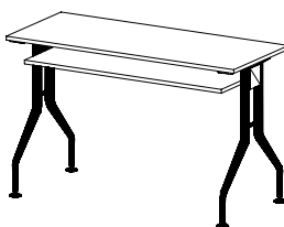
SL 207/18 SL 207/25 školní lavice s pevnou policí / 1350 x 738 x 500 /
