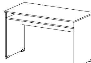
SL 308/18 SL 308/25 školní lavice s pevnou policí / 1350 x 738 x 600 /
