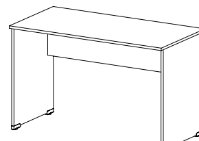
SL 304/18 SL 304/25 školní lavice / 1350 x 738 x 600 /
