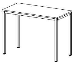
SL 002/18 SL 002/25 školní lavice / 1000 x 738 x 500 /
