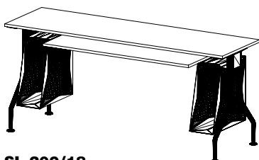
SL 209/18 SL 209/25 školní lavice s pevnou policí a držáky pro PC / 1700 x 738 x 500 /
